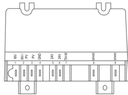
FIGURA 23 - CONTROL DE ENCENDIDO
