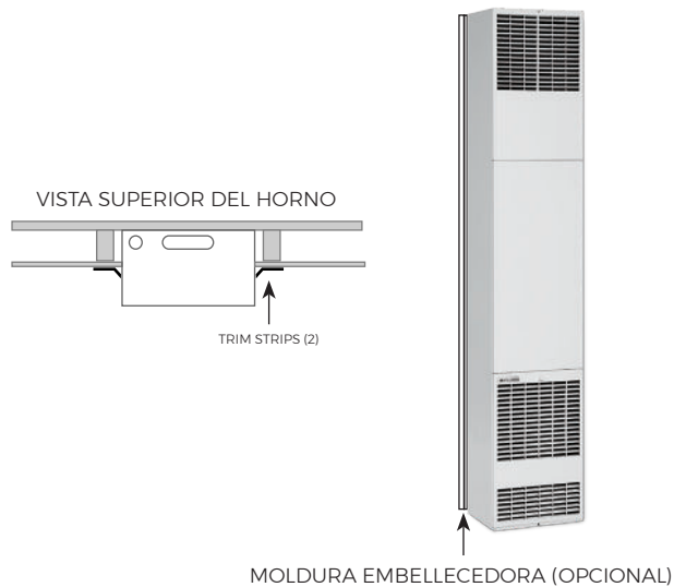
FIGURA 20 - CUERPO DEL CALEFACTOR
