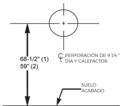
FIGURA 11 - ABERTURA DE PARED (MONTAJE SUPERFICIAL)
