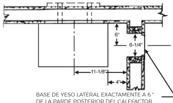
FIGURA 13 - INSTALACION DE LA BASE DE YESO
