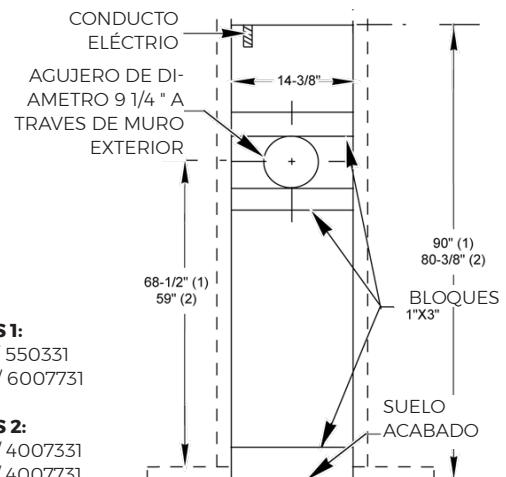
FIGURA 8 - ABERTURA EN LA PARED PARA MONTAJE EMPOTRADO
