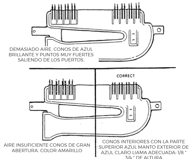
FIGURA 29 - PATRON DE LA LLAMA DEL QUEMADOR PRINCIPAL
