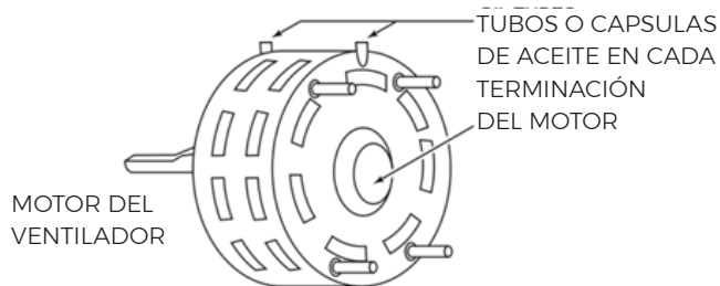
FIGURA 28 - PERFORACIONES DEL MOTOR DE ACEITE
