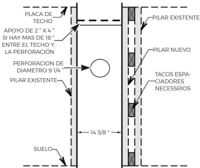
FIGURA 9 - CIERRE DEL ESPACIO DE MONTANTES
