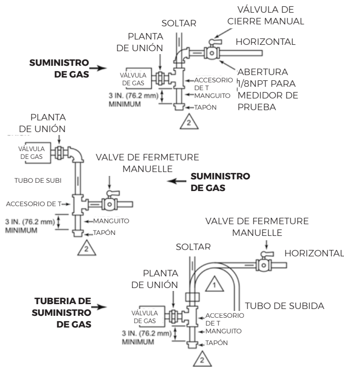
FIGURA 24 - TAMAÑO DE LA TUBERÍA
