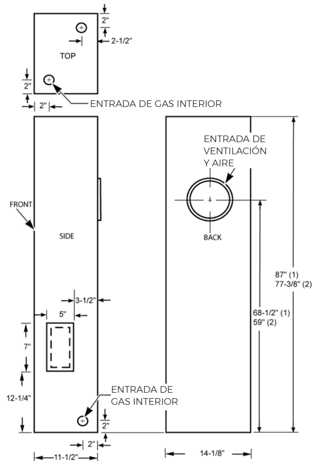
FIGURA 10 - ABERTURAS DE ELECTRICIDAD Y GAS
