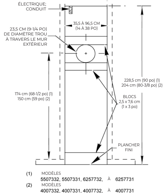
FIGURE 8 - OUVERTURE MURALE POUR MONTAGE ENCASTRÉ
