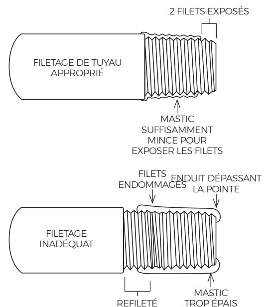
FIGURE 25 - BONNES PRATIQUES EN MATIÈRE DE TUYAUTERIE
