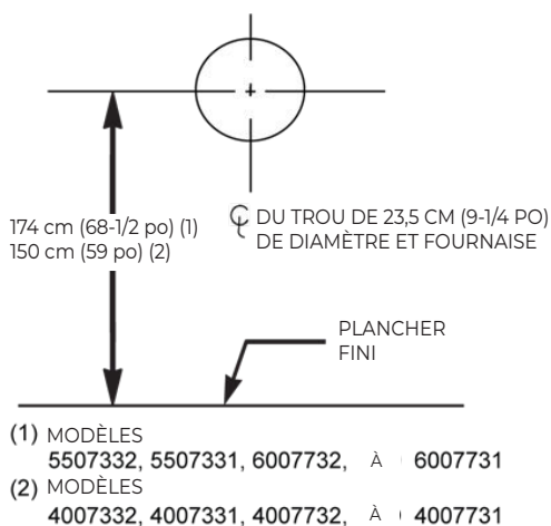
FIGURE 12 - INSTALLATION D'ARRÊT D'ENDUIT
