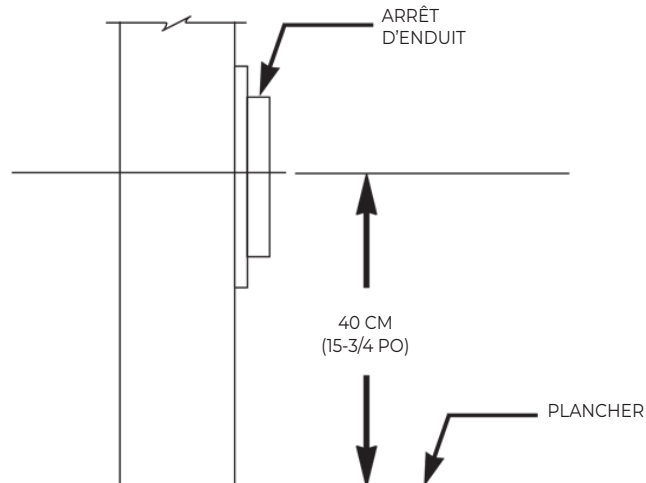
TROSSE DE FIXATION DE LA GRILLE DE SORTIE LATÉRALE EN OPTION N° 6701 Se reporter à la figure 14.
