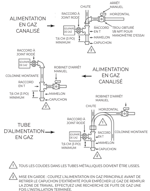
FIGURE 24 - ADMISSION DE GAZ DU CÔTÉ GAUCHE
