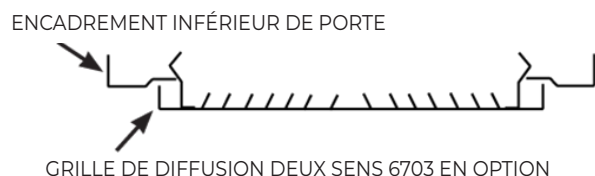
FIGURE 15 - GRILLE DE DIFFUSION DEUX SENS 6703
