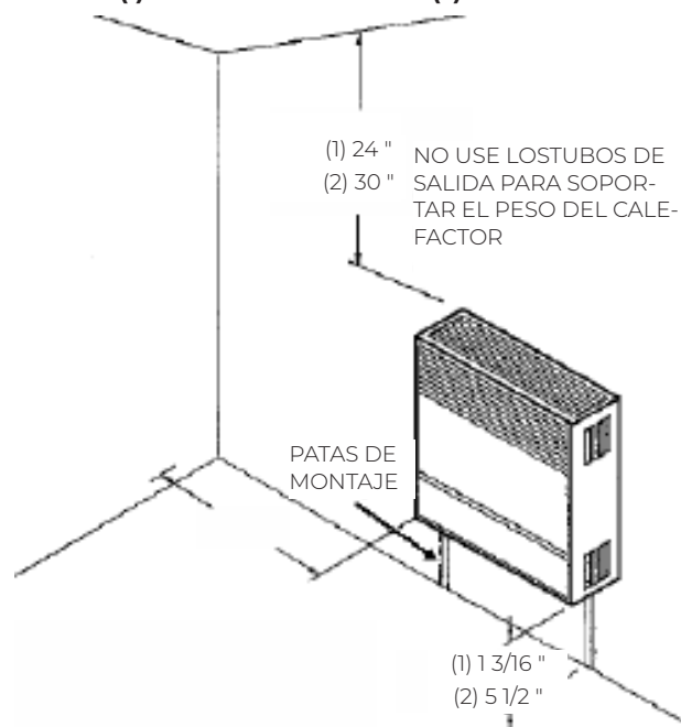
FIGURA 2 - (1) MODELO: SERIE 14038 - (2) MODELO: SERIE 22038
