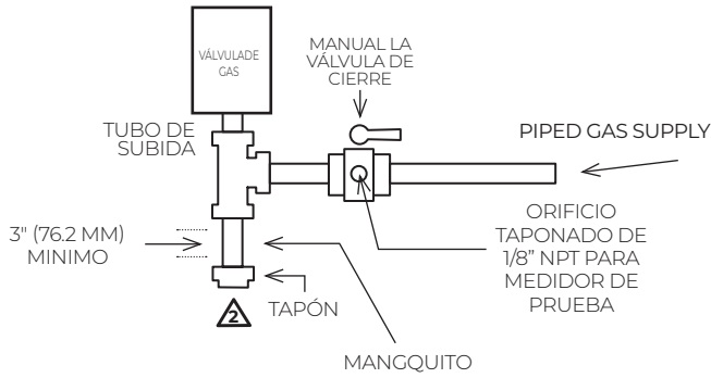
FIGURA 15 – TUBERÍA DE GAS
