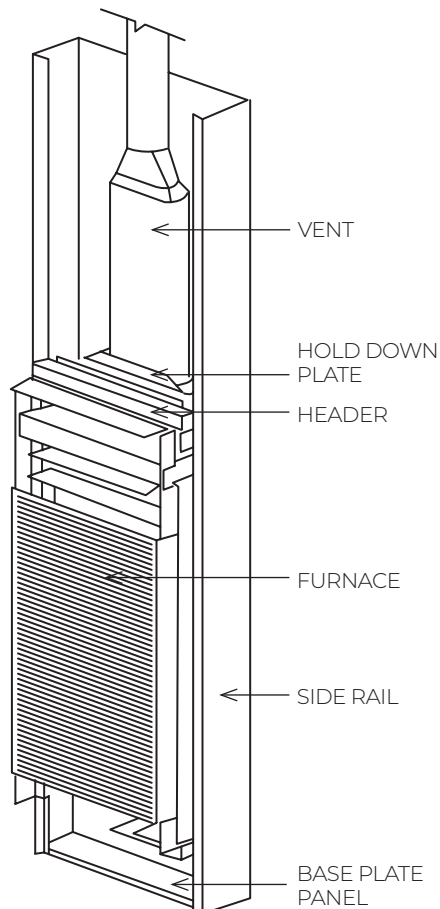
VENTILACIÓN INSTALADA
