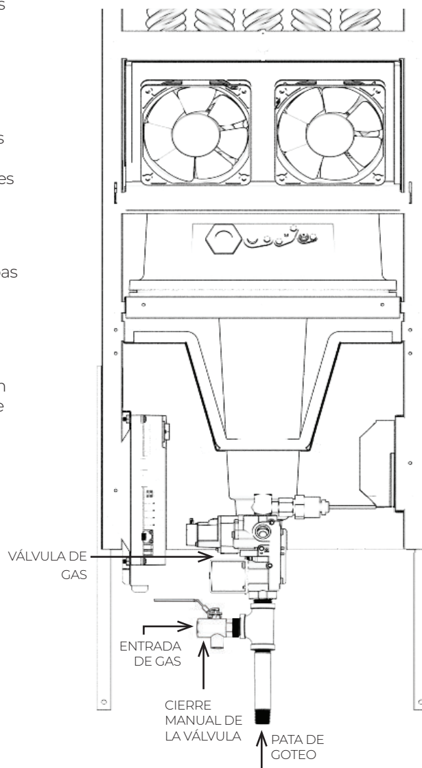
FIGURA 22 – DISCONECTAR LA LÍNEA DE GAS
