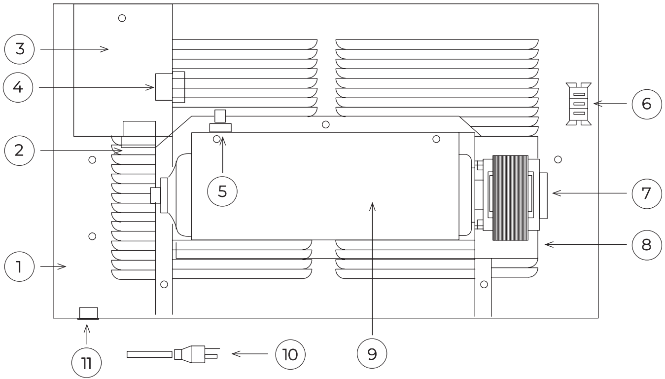
Lista de piezas de repuesto para el registro motorizado trasero – Modelos 6920
