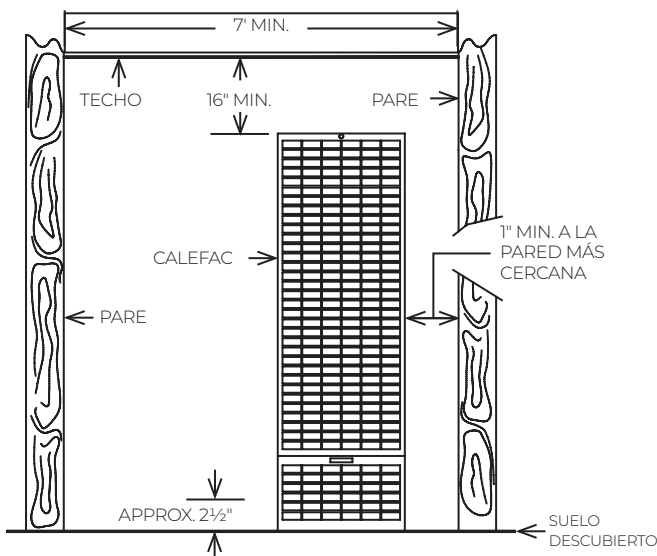
FIGURA 1 – ESPACIO MÍNIMO
