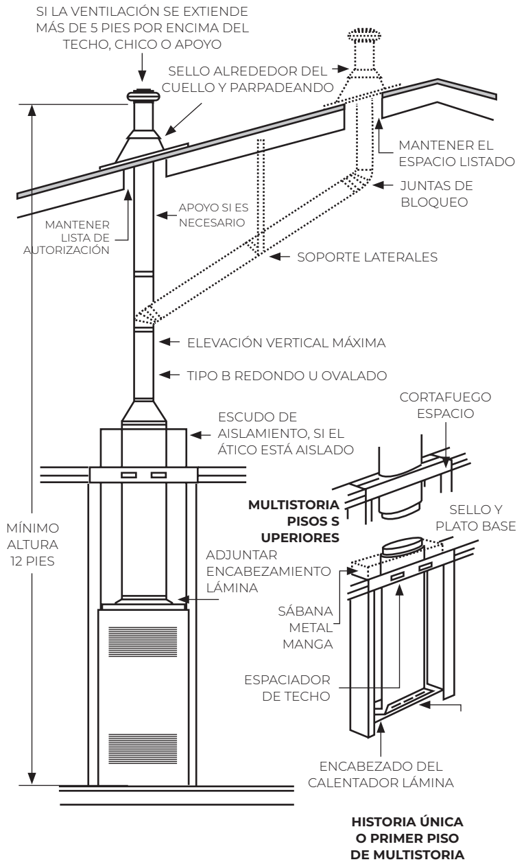
FIGURA 8 – VENTILACIÓN ALTERNATIVA
