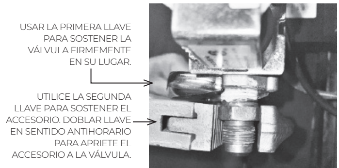
FIGURA 16 - CONEXIÓN DE LA VÁLVULA
