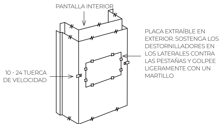
FIGURA B – RETIRAR LAS PLACAS EXTRAÍBLES
