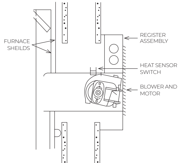
FIGURA 13 – MONTAJE DE ACCESORIO DE VENT. TRASERO
