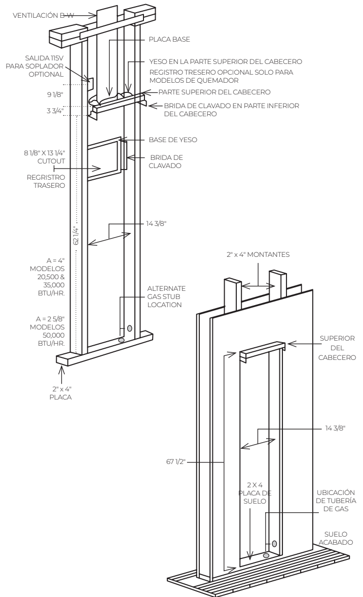
FIGURA 5- INSTALACIÓN DE MONTAJE EMPOTRADO
