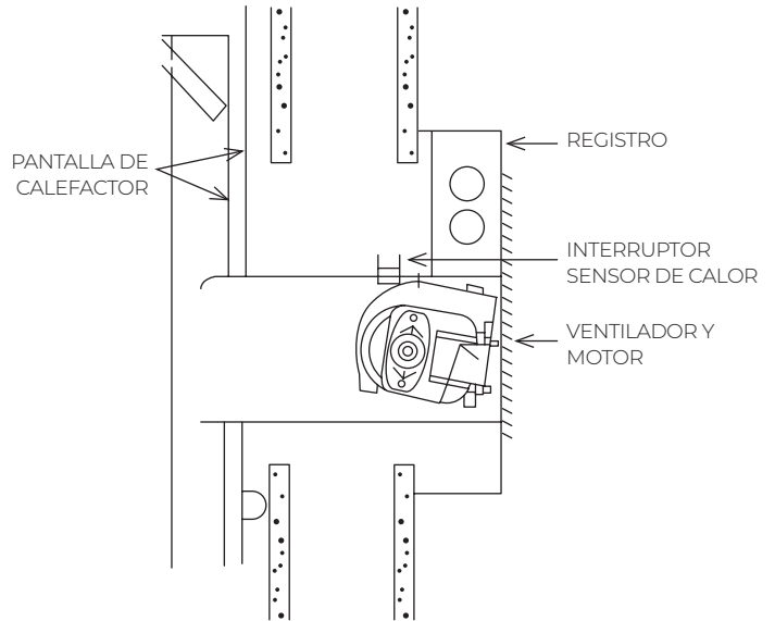
FIGURA C – INSTALACIÓN SUPERFICIAL
