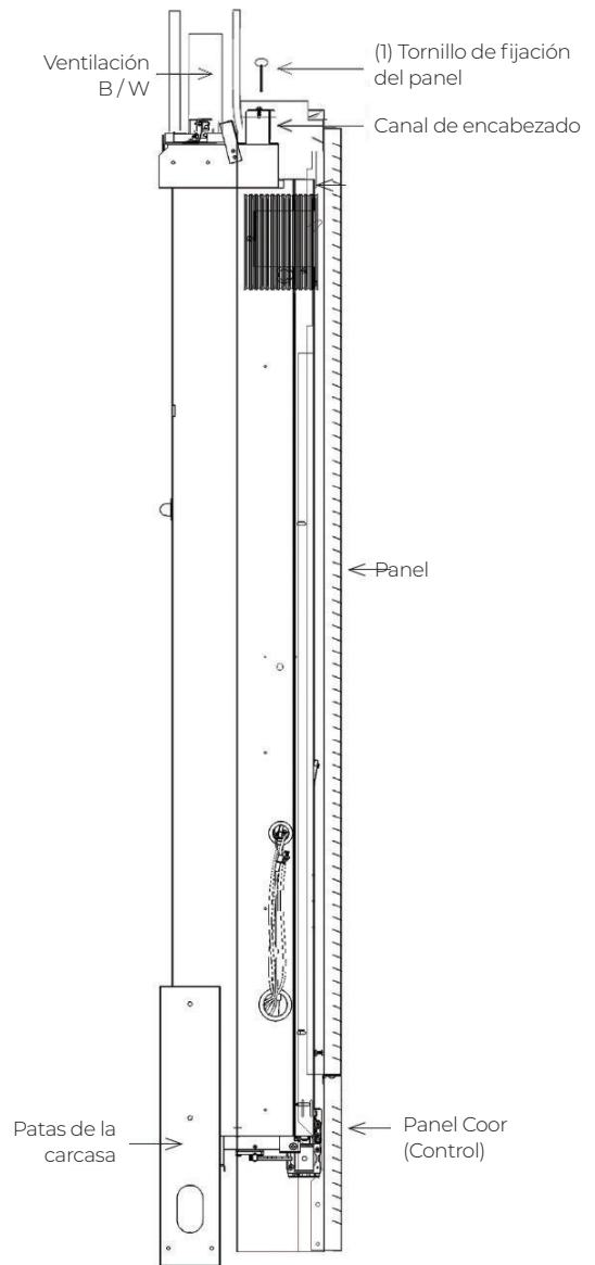
FIGURA 18 – COLOCACIÓN DEL PANEL
