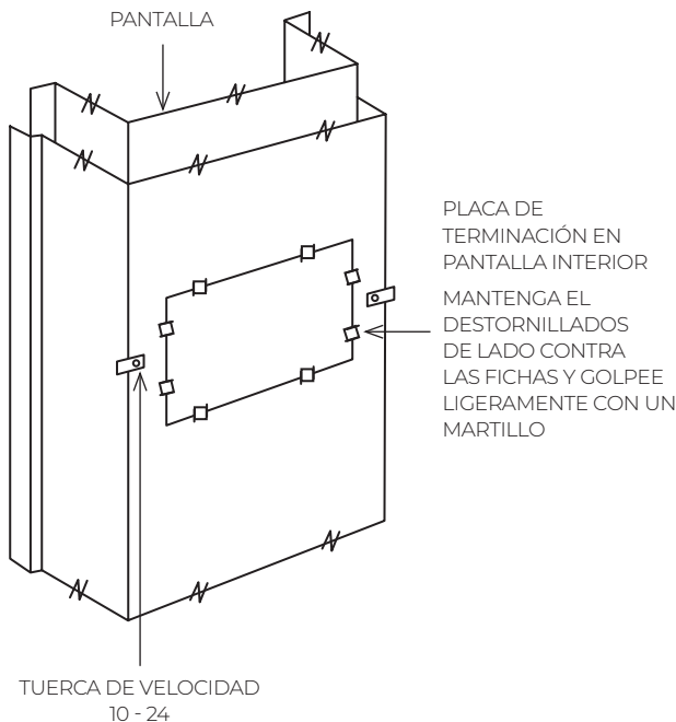
FIGURA 12 – RETIRE LAS PLACAS DE TERMINACIÓN
