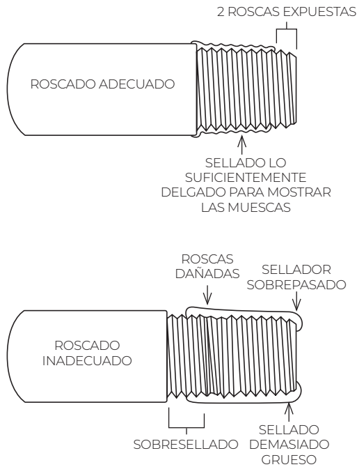
FIGURA 17 – CANALIZACIÓN ADECUADA
