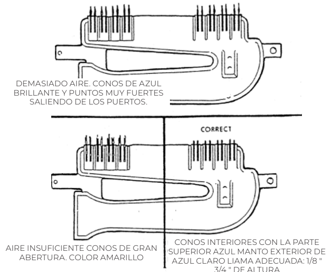
FIGURA 29 - PATRON DE LA LLAMA DEL QUEMADOR PRINCIPAL
